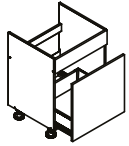
Szafka na wysokość 820 mm (wys. szafki bez blatu)
